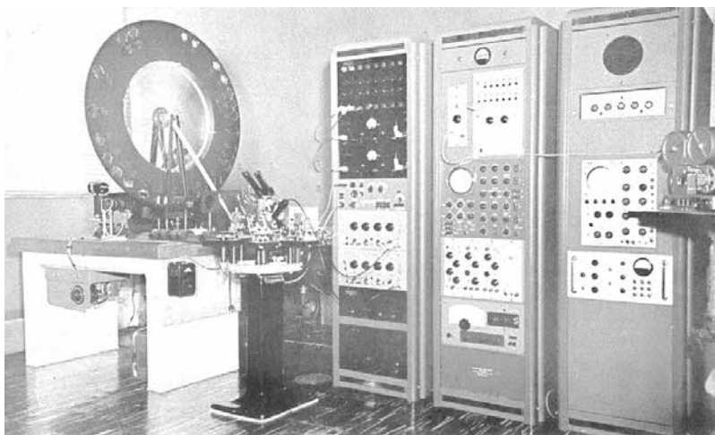
Equipo construido en el IVNIC (1956)
